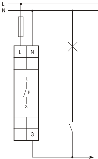
Schéma základního zapojení
